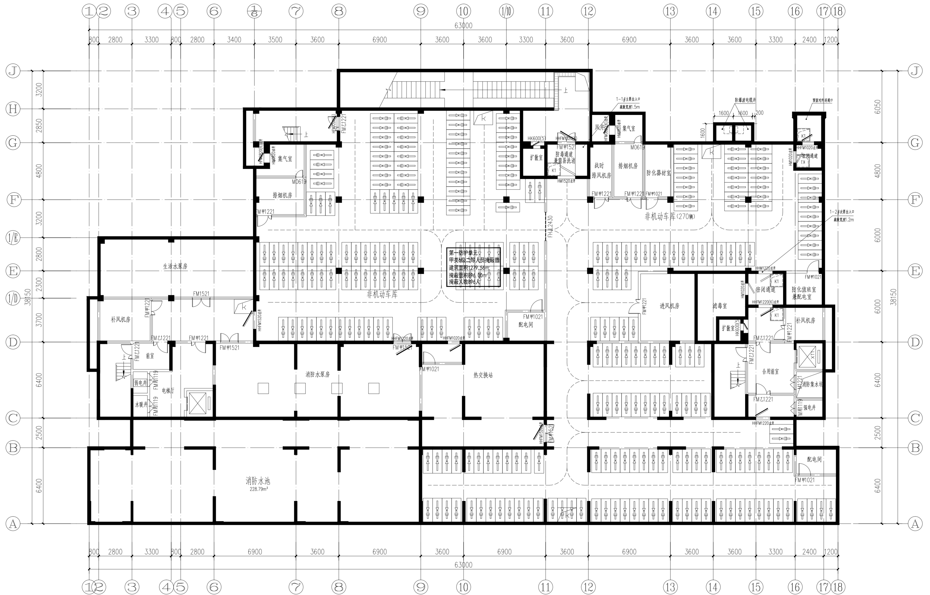
地下一层平面图
